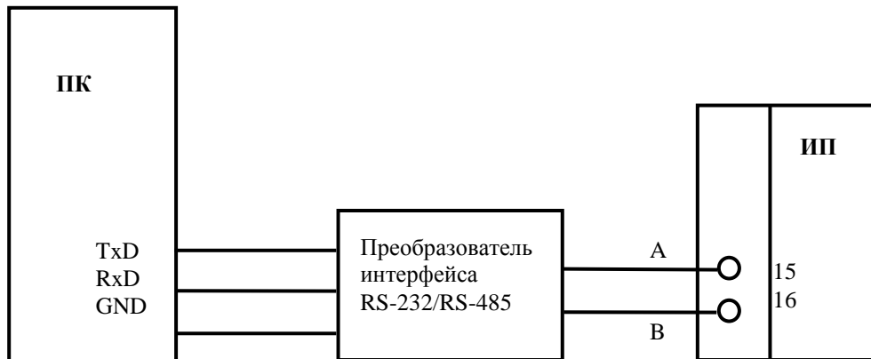
Рисунок 1- Подключение ИП к персональному компьютеру
